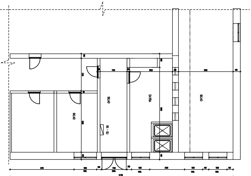
KUCHYNYKA - KD Babín lmp - EXISTUJÚCI STAV
