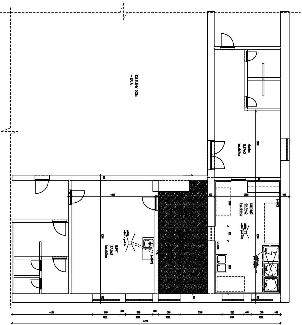
KUCHYNYKA - KD Babín lmp - EXISTUJÚCI STAV
